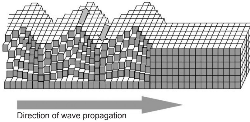
Love wave
